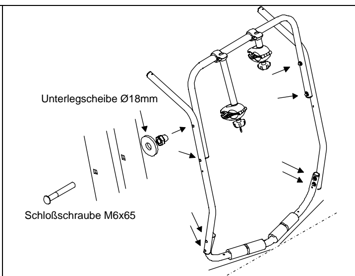
4. Montage der Holme an Trägerrahmen und Querbügel: Achten Sie bei der Montage des Querbügels darauf, dass die Biegung des Querbügels der Kontur der Heckklappe angepasst ist.
