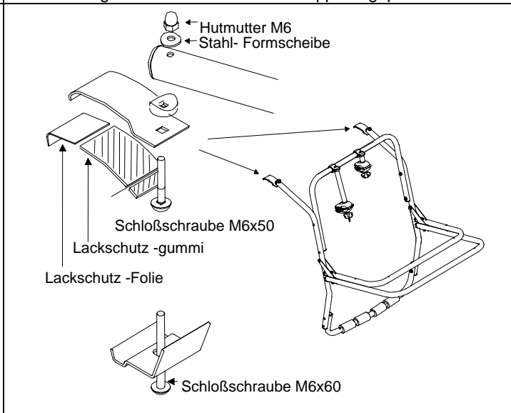
6. Bekleben Sie die oberen Einhängeteile mit den Schutzfolien bzw. Schutzgummis. Evtl. sind die Schutzgummis mit einer Schere zu kürzen. Verschrauben Sie die oberen Einhängeteile an den Trägerholmen.
